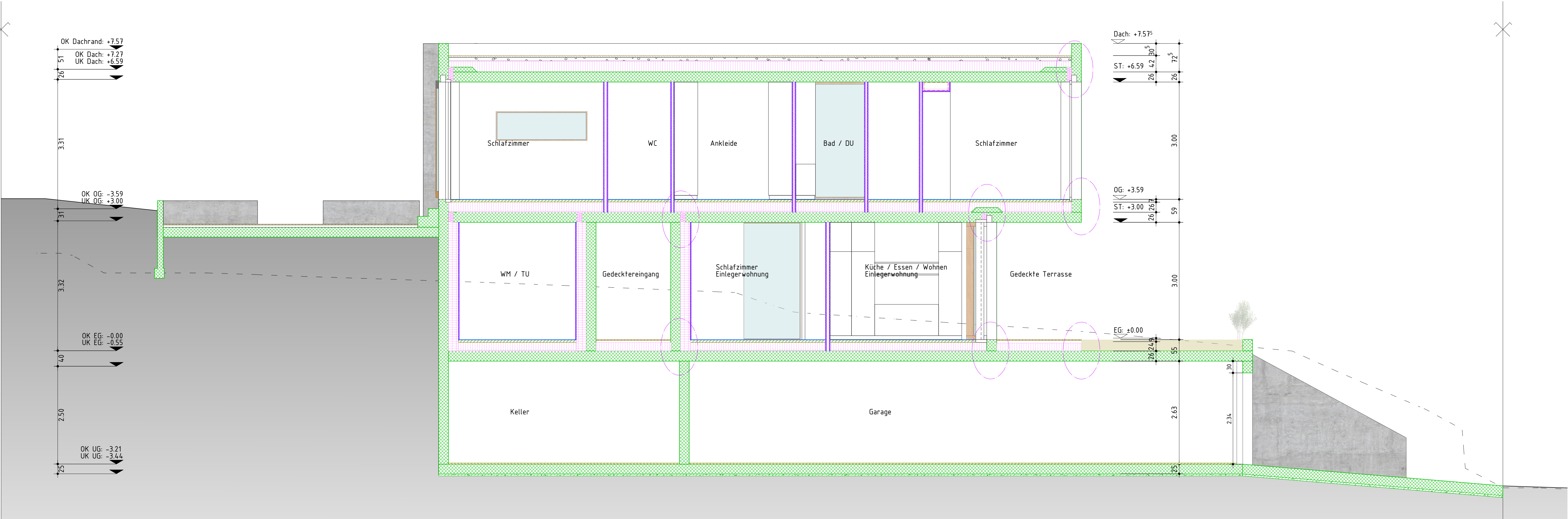
Schnitt D-D
