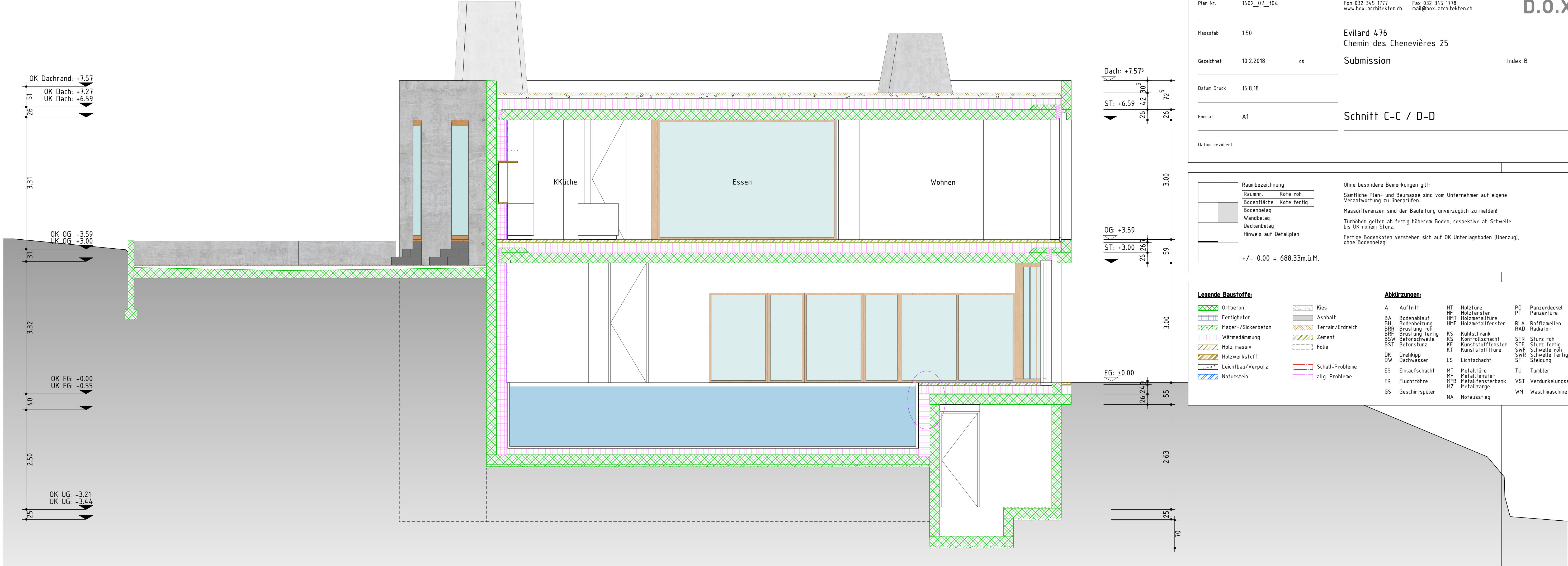
Schnitt C-C
