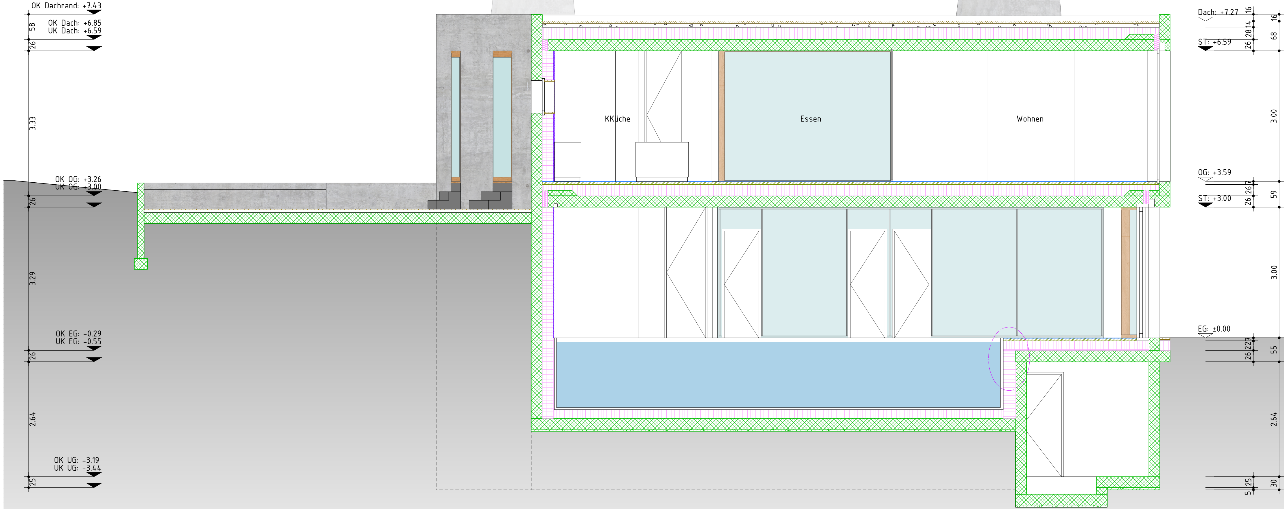
Schnitt C-C
