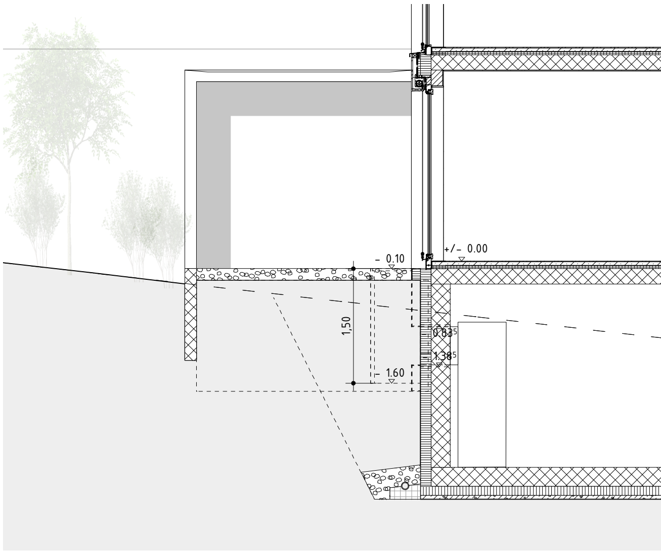
Schnitt
