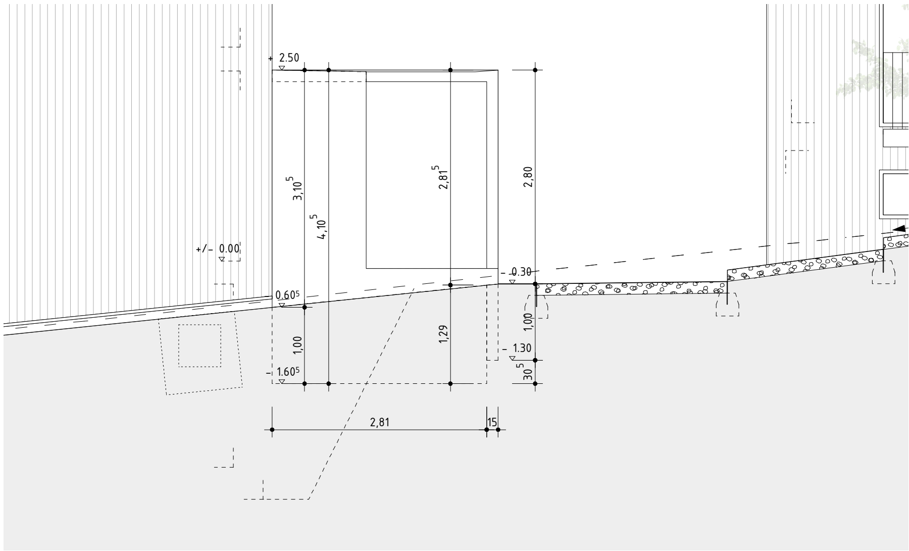
Westfassade
