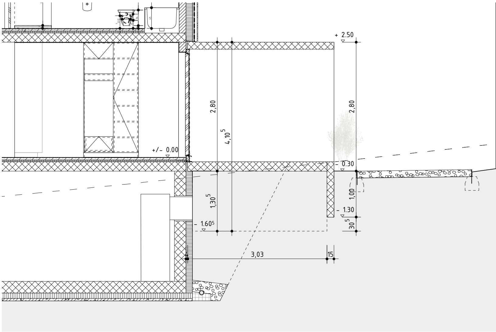
Schnitt
