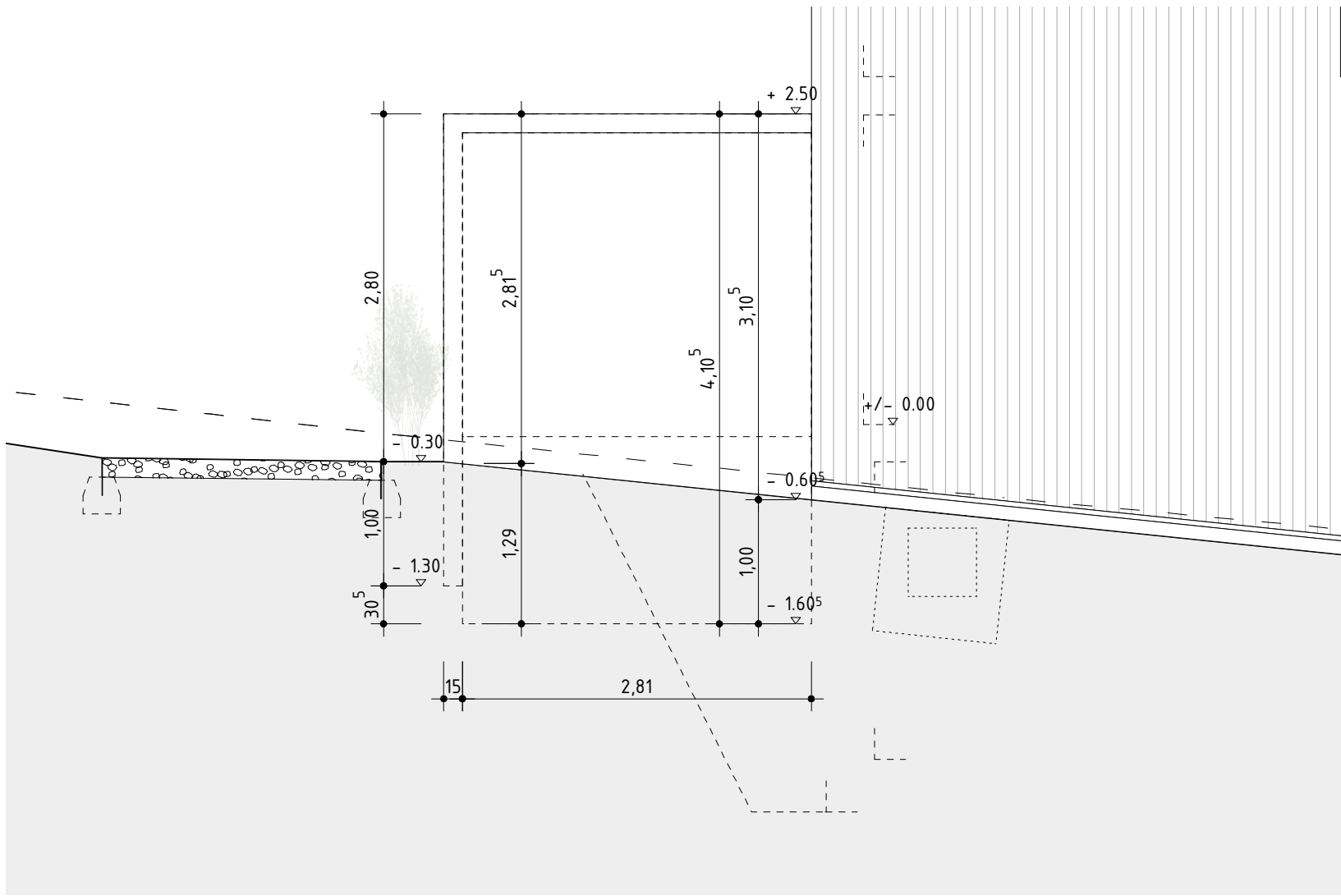
Ostfassade
